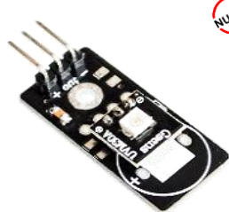
SEN18B 40.000 UVM-30A, Sensor especializado en medir la intensidad de radiación Ultravioleta UV
