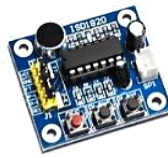
MO21 9.500 ISD1820 Módulo de grabación y reproducción de voz que permite almacenar un mensaje de audio (hasta 10 segundos) y reproducirlo.
