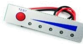
MO44L 8.000 Indicador de nivel de carga visual para paquetes de baterías de litio configurados en serie (2S, 3S o 4S).
