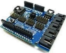
SH04 8.400 Placa expansora para sensores y motores, funcional porque duplica los pines para más conexiones.
