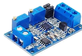
MO67A 3.200 Módulo de voltaje 4-20mA a 0-10v transmisor de voltaje convertidor señal
