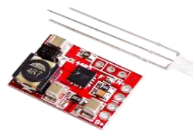
MO44C 3.000 TP5000 es un módulo de carga, cargador de tipo conmutado (Switching) con led indicador.
