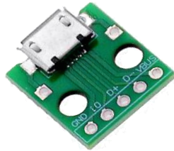
MO07C-1 - USB V8 de montaje para PCB o prototipado para alimentar tus proyectos o transferir datos.
