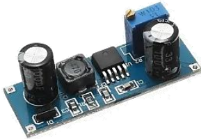
MO42B-3 4.300 XL7015 Modulo regulador de voltaje Entrada: 5-80v Salida: 5-20v 1amp
