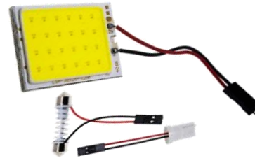
LED COB de alta potencia 28v -34v
