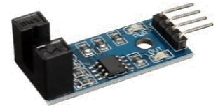
SEN17 3.200 Sensor optico de velocidad infrarrojo
